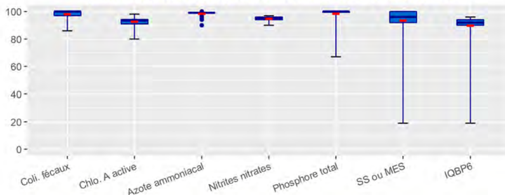
IQBP6 et ses sous-indices à la station 04310008 de la rivière des Outaouais à TNO aquatique de la MRC de Pontiac calculés pour les périodes estivales comprises entre mai 2001 et octobre 2021
