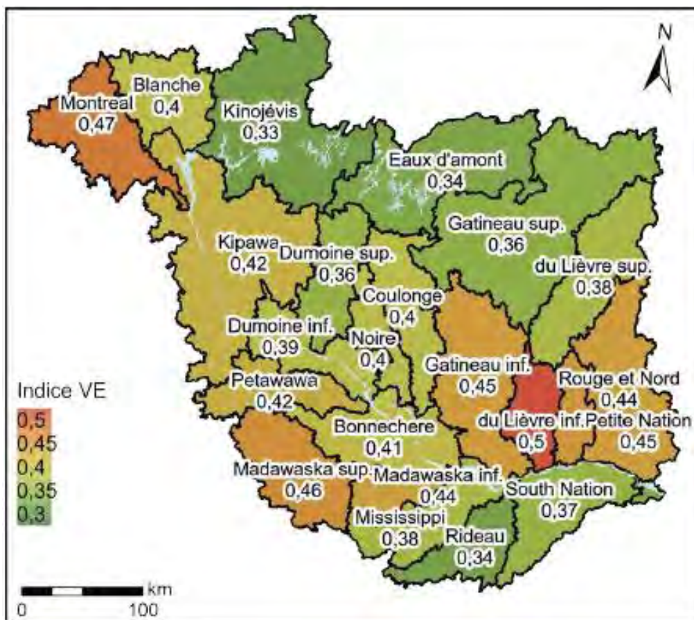
Figure 4-5. Indice pondéré et standardisé de vulnérabilité environnementale, moyenné spatialement pour chacun des sous-bassins versants du bassin versant de la rivière des Outaouais
